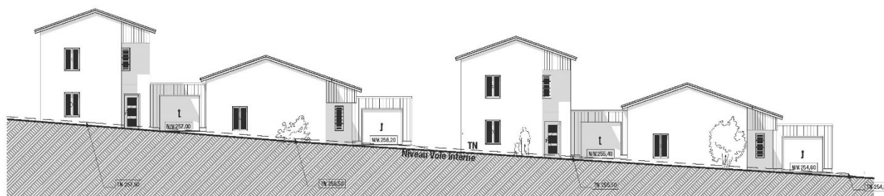
ELEVATION NORD EST LOGTS 1 à 4
